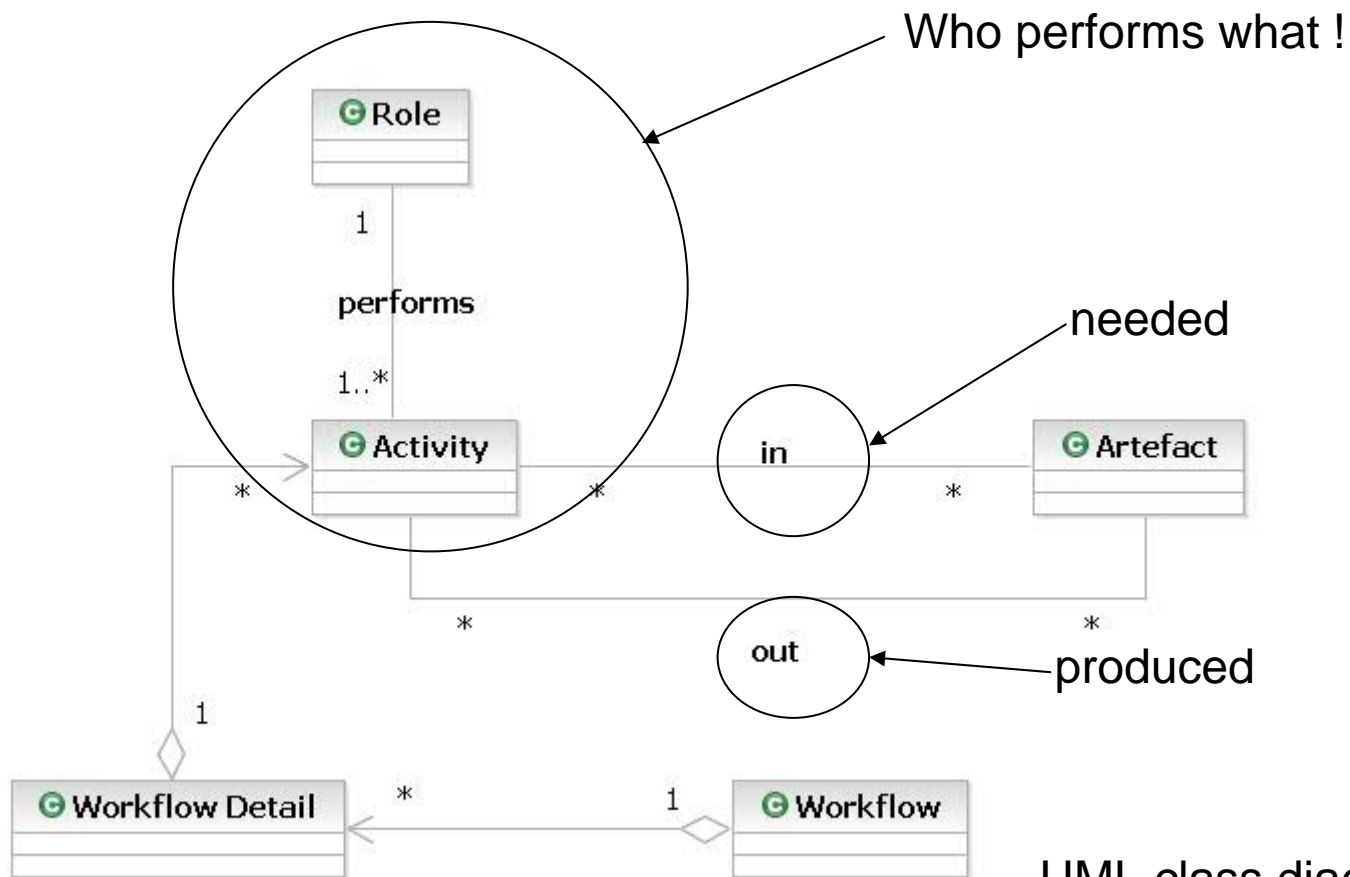
UML class diagramme
